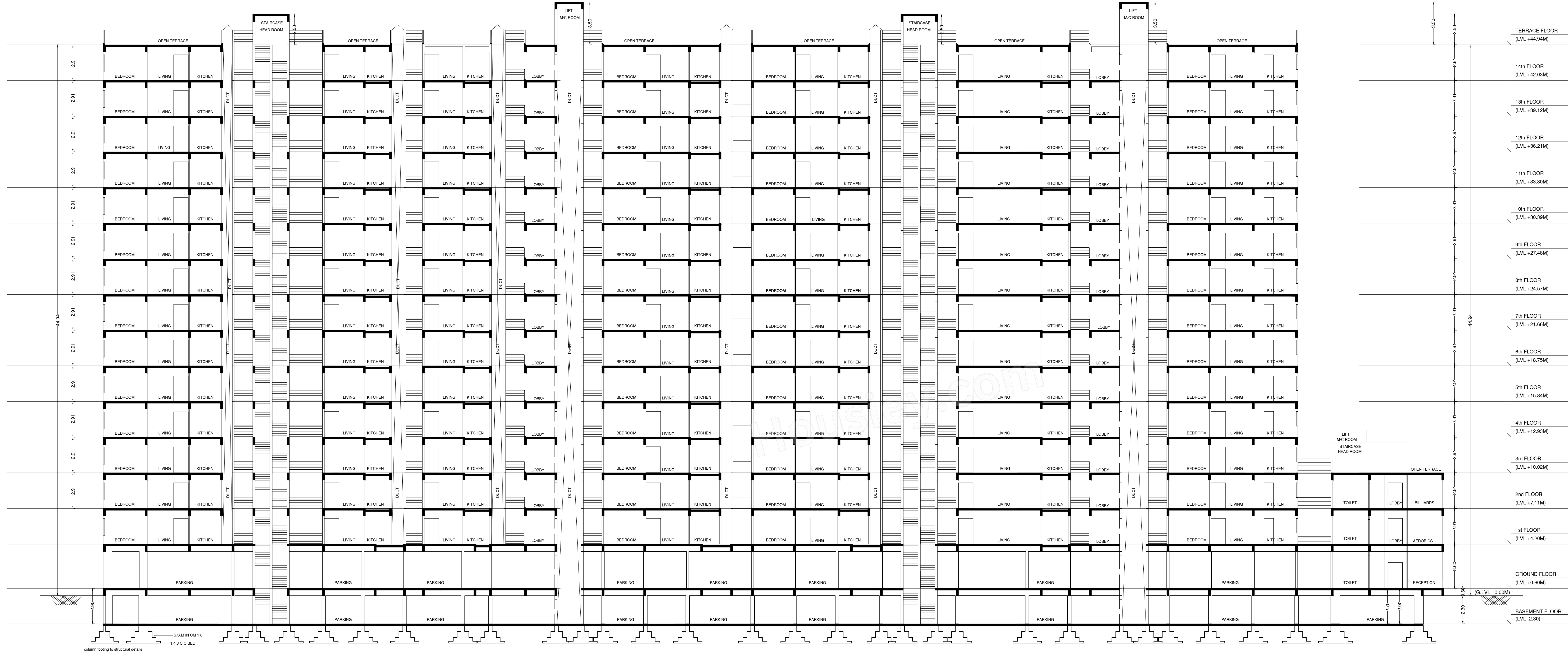
SECTION A-A
